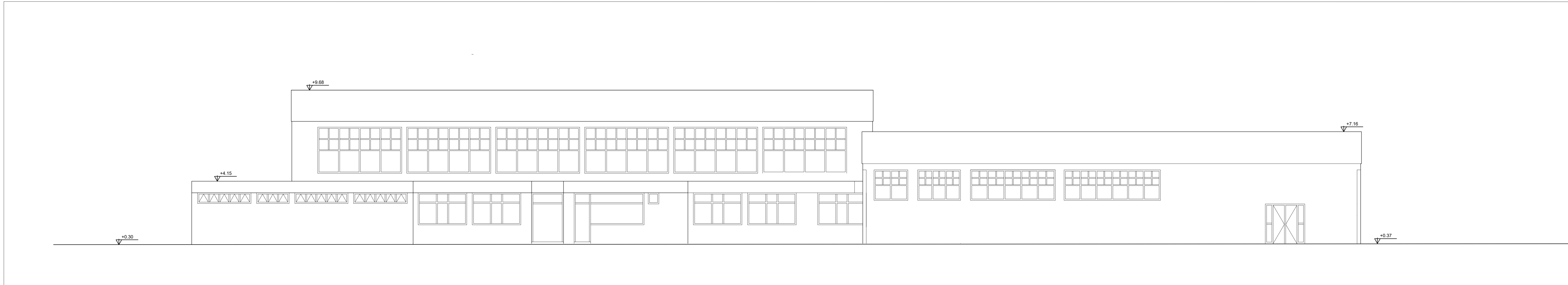
Sezione Ovest - scala 1:100
